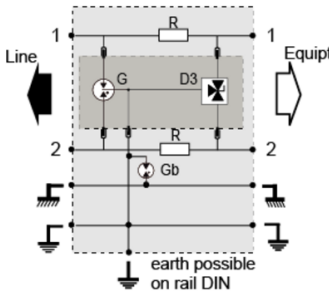
G: 3-электродная газовая трубка Gb: 2-электродная газовая трубка R: резистор D: фиксирующий диод
